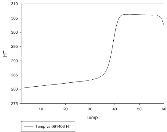
091406 m \Delta F NBD1Tmelt
